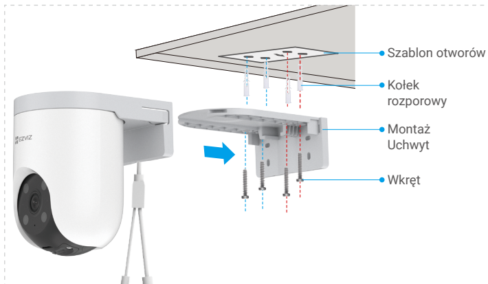
Rys. 1 Montaż sufitowy
